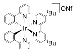
光触媒
