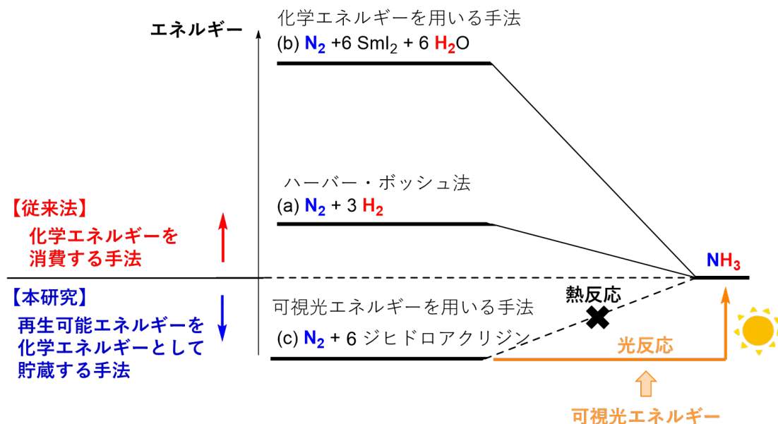
図2 アンモニア合成のエネルギー変化図
