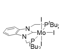
触媒
